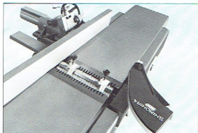
●クシ形口金採用により騒音低下。 ●マグネット式セッティングゲージで刃物セットは簡便。
