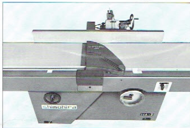
●複式扇形安全カバーを装置しております。 ●使い易い機械前面。
